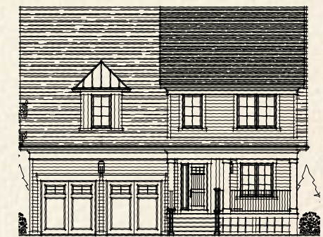
Elevation B
